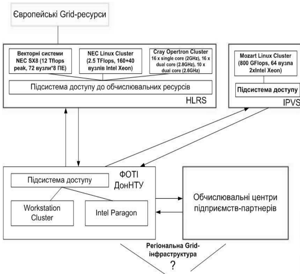
Рисунок 1 – Апаратно-системне забезпечення РПМС
