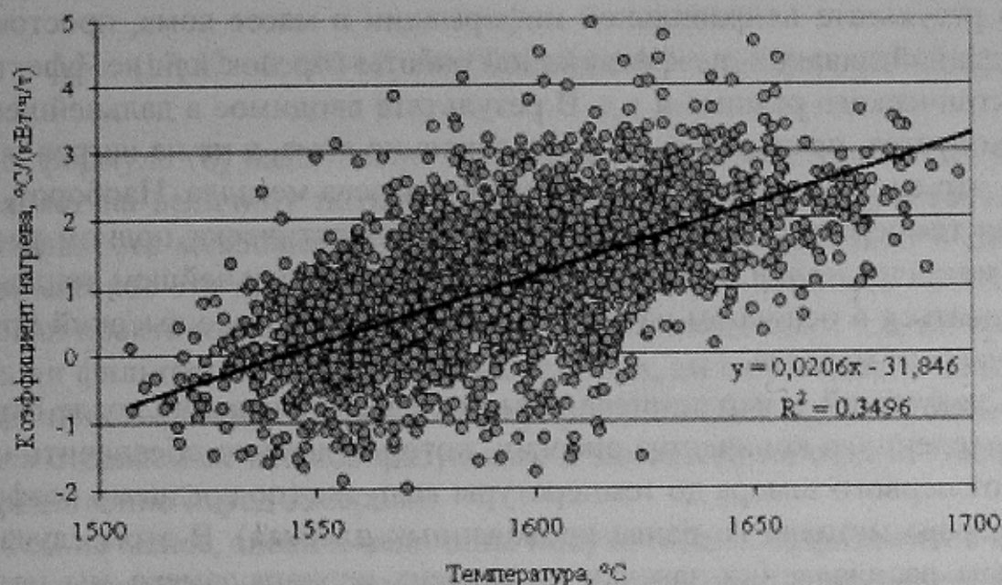
Рисунок 2 – Зависимость коэффициента нагрева металла от конечной температуры ( T_2 ).
