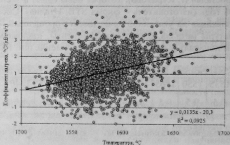
Рисунок 1 – Зависимость коэффициента нагрева металла от средней температуры ( T_{cp} ).
