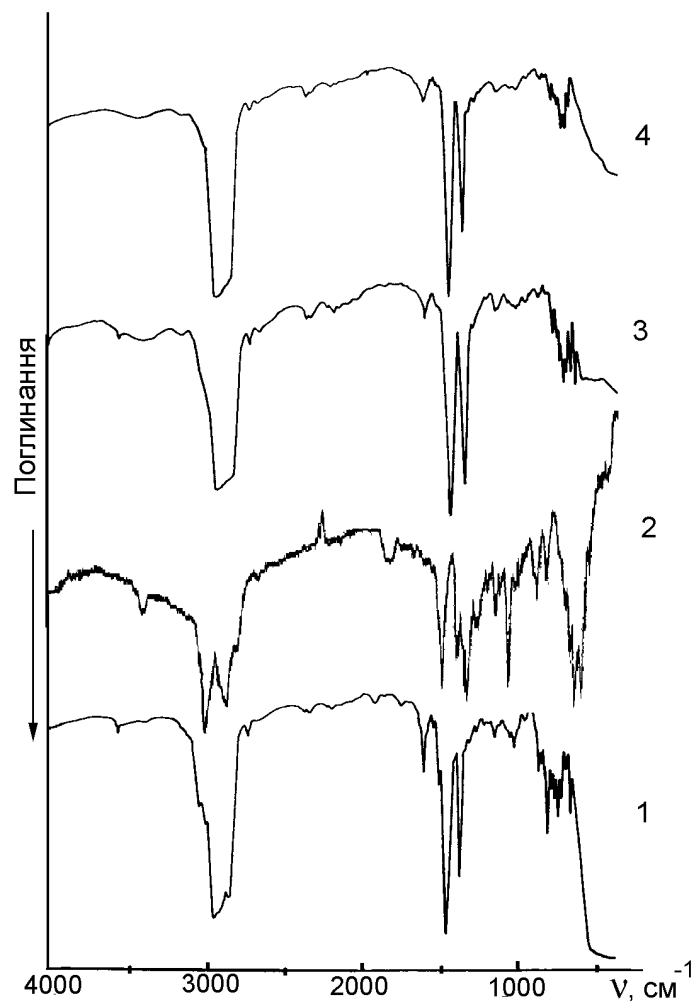
Рис.3 ІЧ-спектри реагентів-збирачів: 1- флотореагент ААР-2; 2 - коксохімічний флотореагент УР-410; 3 – гас; 4 – дизельне паливо.
