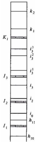
Рисунок 7.1. До приклада знаходження ліній обріза вугільного пласта з розривним тектонічним порушенням та побудови гіпсометричного плану його підосви
