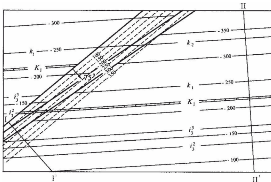
Рисунок 7.2. Приклад первинних графічних побудов для знаходження ліній обріза вугільного пласта i_3 з розривним тектонічним порушенням та побудови гіпсометричного плану його підосви
