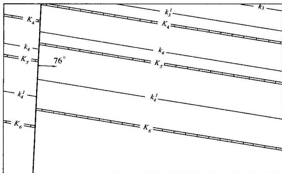
Рисунок 7.7. Завдання на знаходження ліній обрізу вугільних пластів з розривним тектонічним порушенням та побудову гіпсометричних планів їх підосви.
