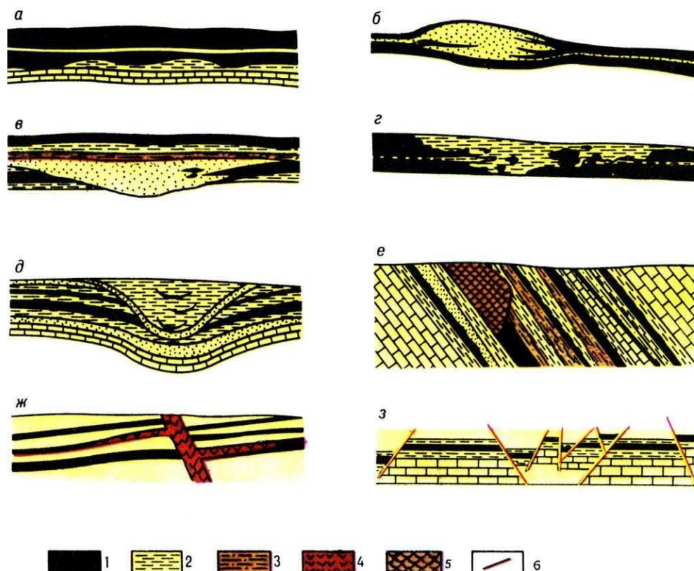
Рисунок 1.3. Ускладнення морфології і залягання вугільних пластів в результаті: а - нерівностей ложа торфовища; б - впровадження у вугілля піщаників; г - розмивів (Кузбас, Донбас); д - карстових просідань в породах, що підстилають вугленосні відкладення; е - вигорання вугілля з утворенням так званих «горельників»; ж - впровадження магматичних тіл; з – з мілкоамплитудною тектонічною порушеністю (Донбас); 1-вугілля, 2 - глина, 3 - алевроліт, 4 - магматичні породи, 5 – «горельники», 6 - розривні порушення.
