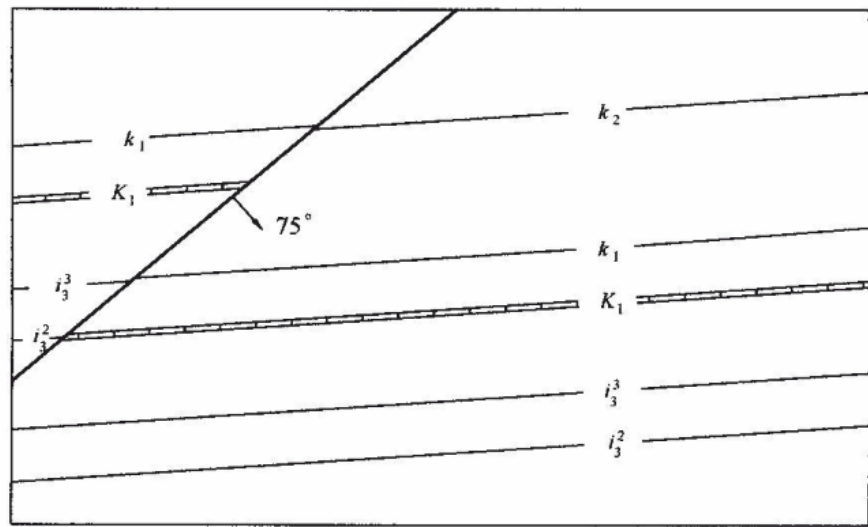
Рисунок 7.1. До приклада знаходження ліній обріза вугільного пласта з розривним тектонічним порушенням та побудови гіпсометричного плану його підосви
