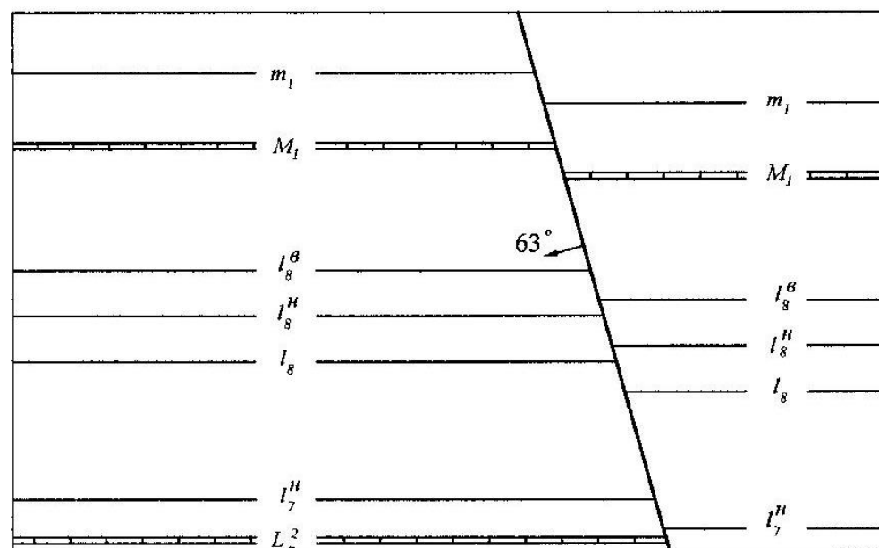
Рисунок 7.9. Завдання на знаходження ліній обрізу вугільних пластів з розривним тектонічним порушенням та побудову гіпсометричних планів їх підосви.
