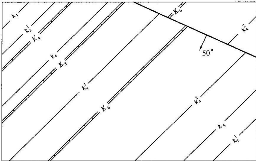
Рисунок 7.5. Завдання на знаходження ліній обрізу вугільних пластів з розривним тектонічним порушенням та побудову гіпсометричних планів їх підосви
