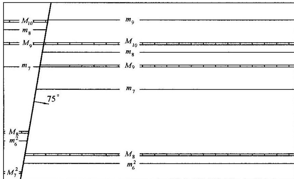
Рисунок 7.8. Завдання на знаходження ліній обрізу вугільних пластів з розривним тектонічним порушенням та побудову гіпсометричних планів їх підосви.
