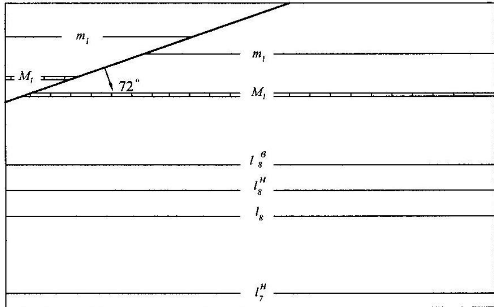
Рисунок 7.10. Завдання на знаходження ліній обрізу вугільних пластів з розривним тектонічним порушенням та побудову гіпсометричних планів їх підосви.
