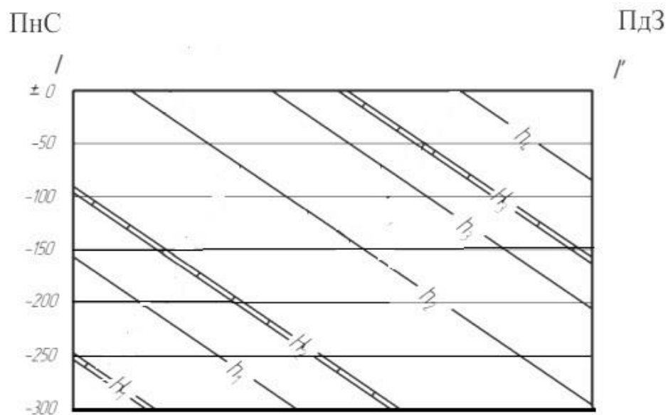
Рисунок 3.2. Приклад побудов геологічного розрізу до геологічної карти вздовж лінії I-I'
