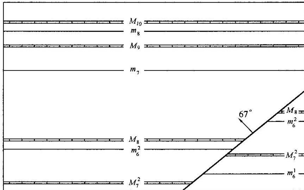
Рисунок 7.6. Завдання на знаходження ліній обрізу вугільних пластів з розривним тектонічним порушенням та побудову гіпсометричних планів їх підосви.
