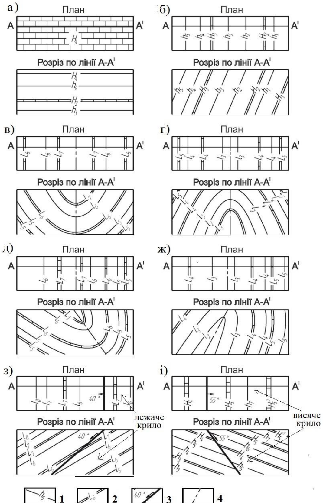
Рисунок 4.1. Основні форми залягання гірничих порід, морфологічні типи складок та розривних порушень Донбасу:
