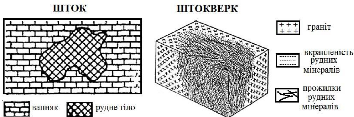
Рисунок 1.1. Ізометричні форми тіл корисних копалин
