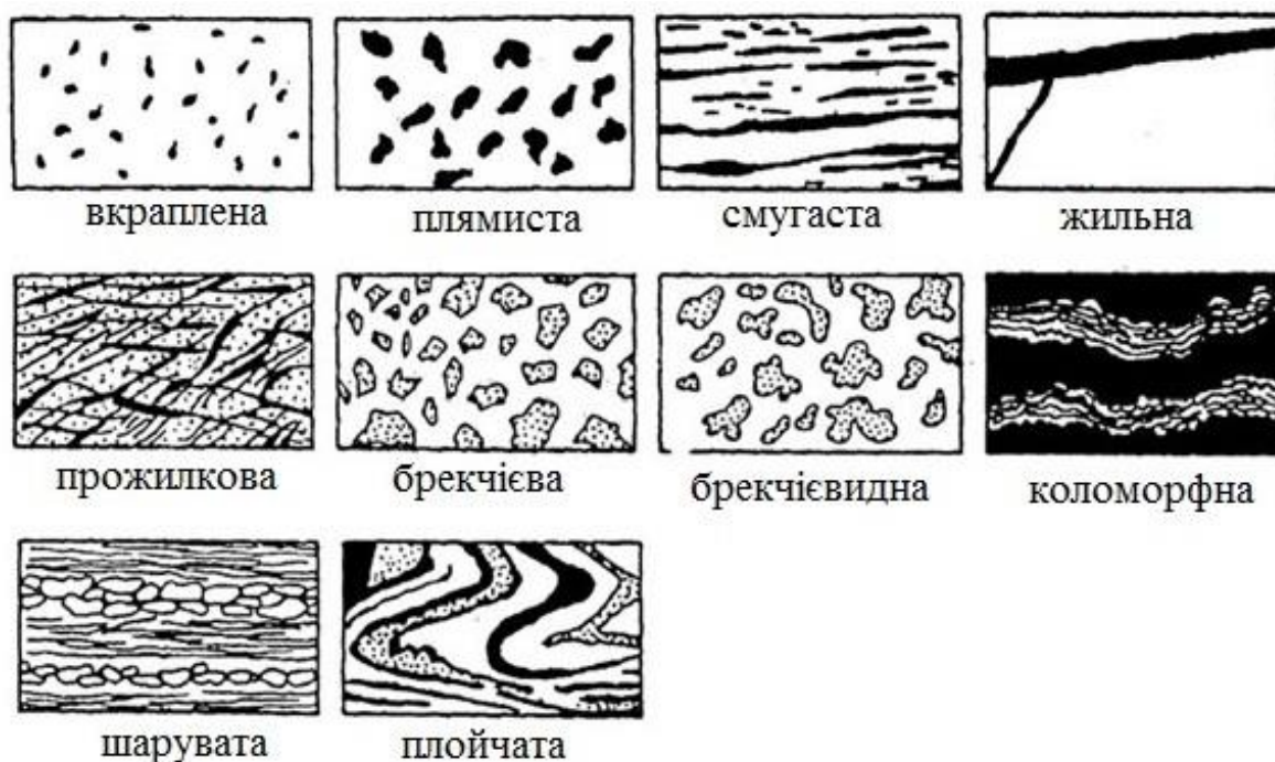
Рисунок 1.4. Головні типи текстур корисних копалин
