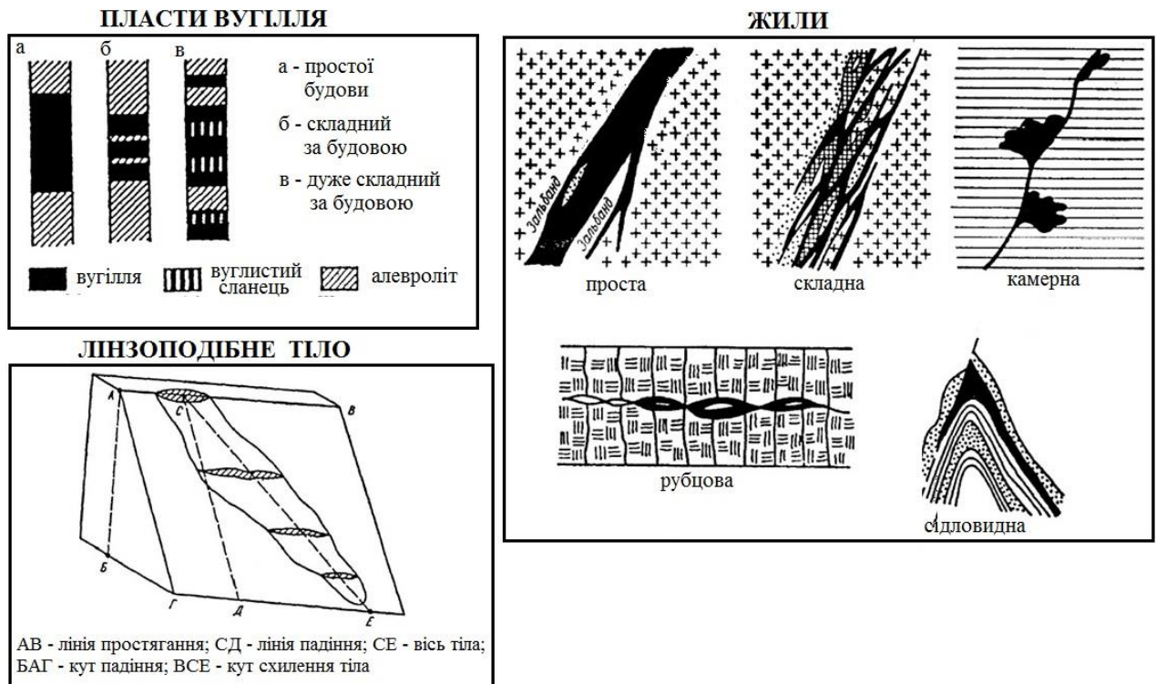
Рисунок 1.2. Схематична будова плитоподібних форм тіл корисних копалин
