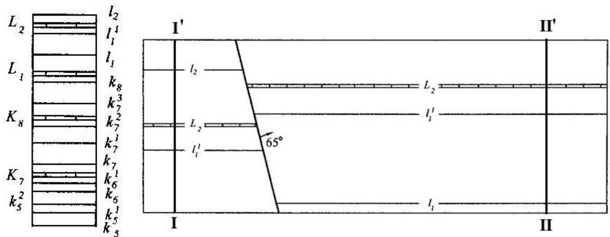
Рисунок 3.3. Геологічна карта ділянки шахтного поля Донецько-Макіївського вугленосного району масштабу 1:5 000 для виконання 3 завдання практичної роботи
