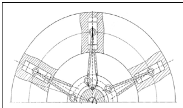
Рис. 3. Конструкция маховика с массивными ползунами
