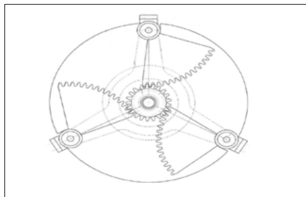
Рис. 2. Конструкция маховика с трехлучевым кронштейном
