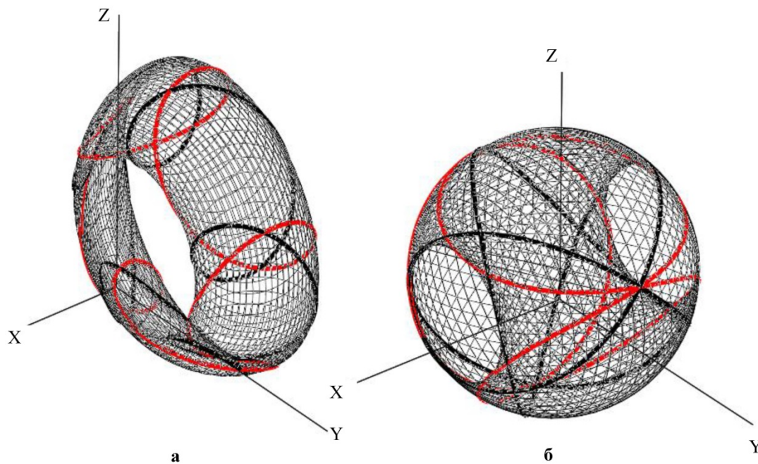
Рис. 3. Вигляд траскторій руху одиничного робочого інструменту та поверхні-носія при двох обертових рухах за додавальною та різницевою схемами роботи виконавчого органу (а – у загальному випадку, б – при сферичному русі)
