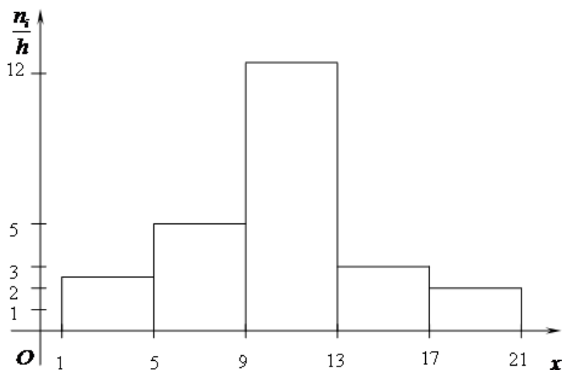
Рисунок 5.2 – Гістограма частот
