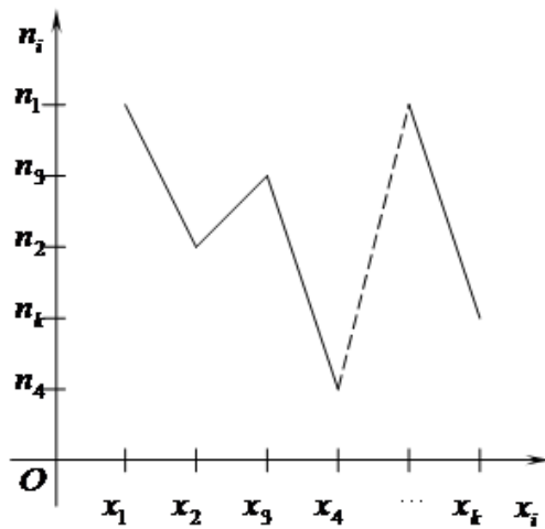
Рисунок 5.1 – Полігон частот
