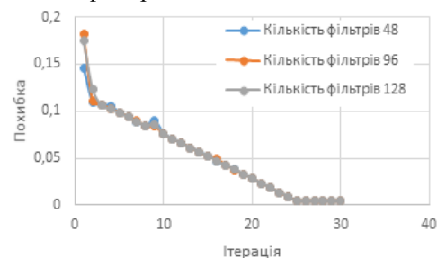
Рисунок 6 – Вплив кількості фільтрів на похибку при навчанні мережі
