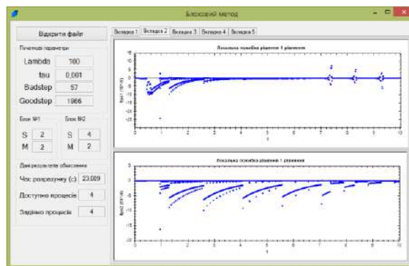
Рисунок 9 – Графіки локальної похибки для 1 та 2 рівнянь системи
