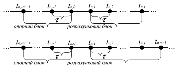
Рисунок 1 – Схема блокового методу зі збільшеним розрахунковим блоком
