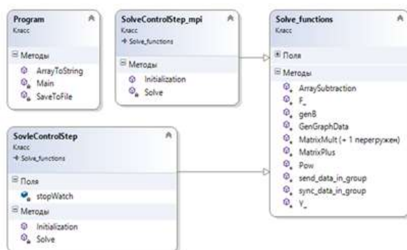
Рисунок 5 – Діаграма класів
