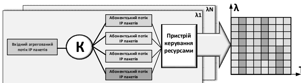
Рис. 6 – Функціональна модель вихідного каскаду крайового вузла OBS мережі
