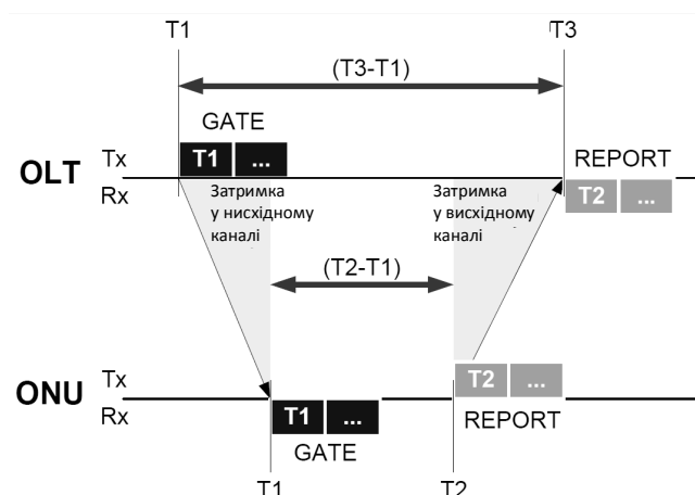
Рисунок 1 – Протокольна діаграма взаємодії OLT та ONU.
