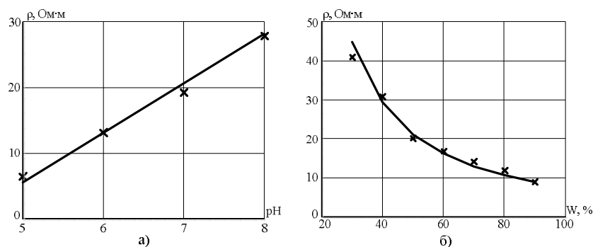
Рисунок 2 – Результат експериментальних досліджень: а) – залежність УЭС почвы от рН при вологості – 60 %; б) – залежність УЭС почвы от вологості при рН – 7 ед.
