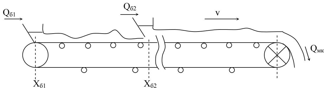
Рисунок 2 – Магістральний стрічковий конвеєр з двома пунктами навантаження
