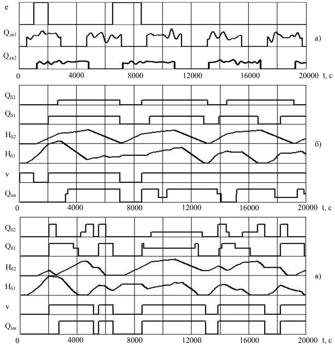
Рисунок 4 – Результати моделювання стану розгалуженої конвеєрної лінії (а – стан магістрального конвеєра і дільничі (вхідні) вантажопотоки, б – стан елементів транспортної лінії за відсутності керування з метою стабілізації, в – стан елементів транспортної лінії в режимі стабілізації вихідного вантажопотоку)
