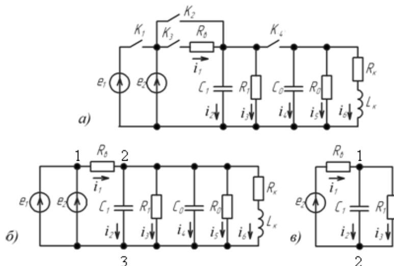
Рисунок 4 - Схеми заміщення мережі: а – універсальна для всіх етапів аварійного процесу; б – в момент виникнення витоку струму на землю; в – після відключення контактора відгалуження з витоком
