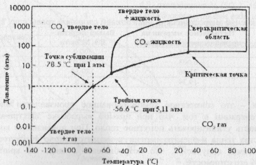
Рис. 2. Фазовая диаграмма равновесий углекислоты в зависимости от температуры и давления
