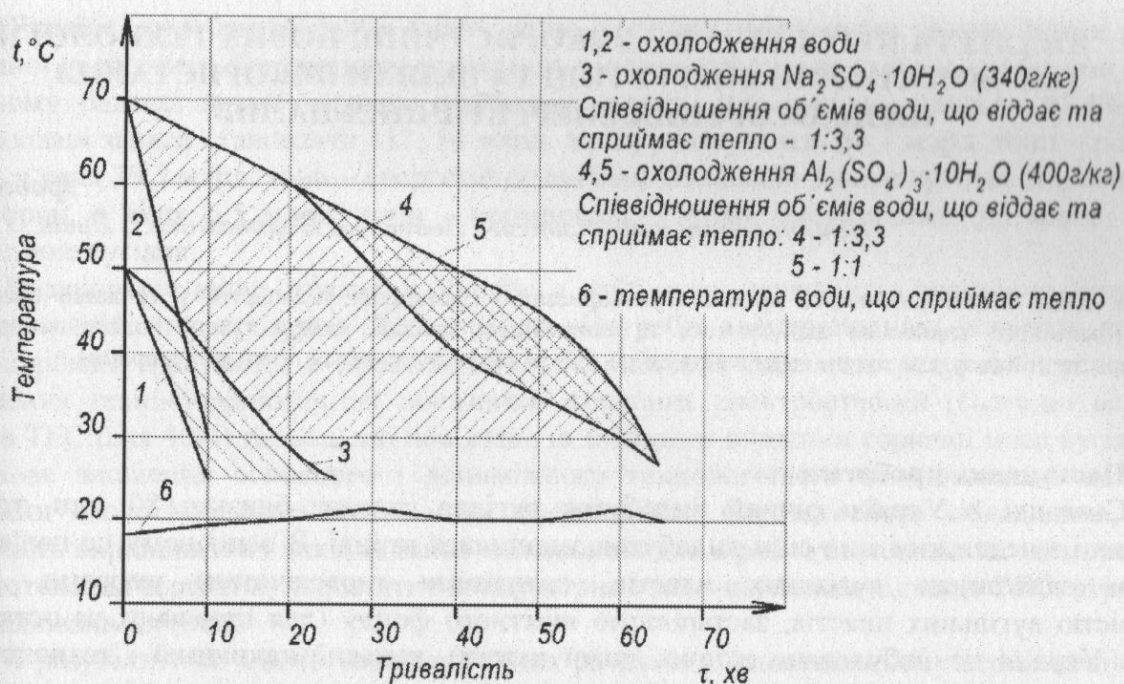
Рис. 3. Сравнительная характеристика аккумуляирования тепла сульфатом алюминия ( \text{Al}_2(\text{SO}_4)_3 \cdot 18\text{H}_2\text{O} ) и сульфатом натрия ( \text{Na}_2\text{SO}_4 \cdot 10\text{H}_2\text{O} )
