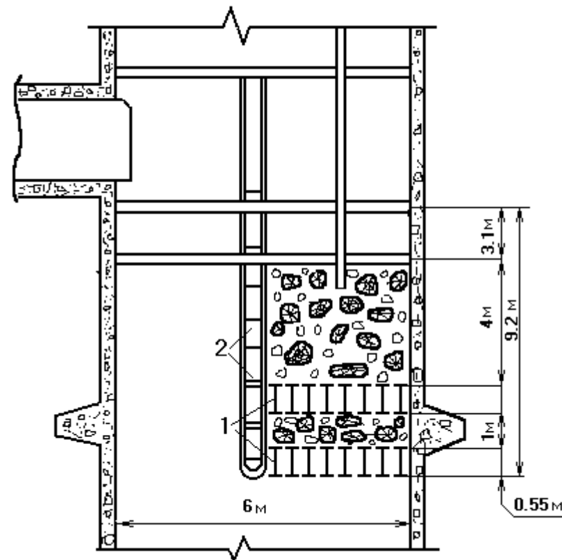
Рисунок 1.5 - Конструкция полка
