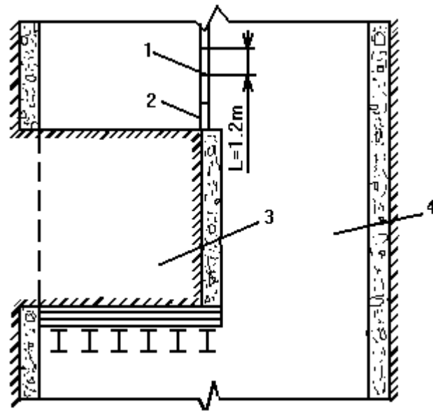
Рисунок 1.6 - Схема отшивки
