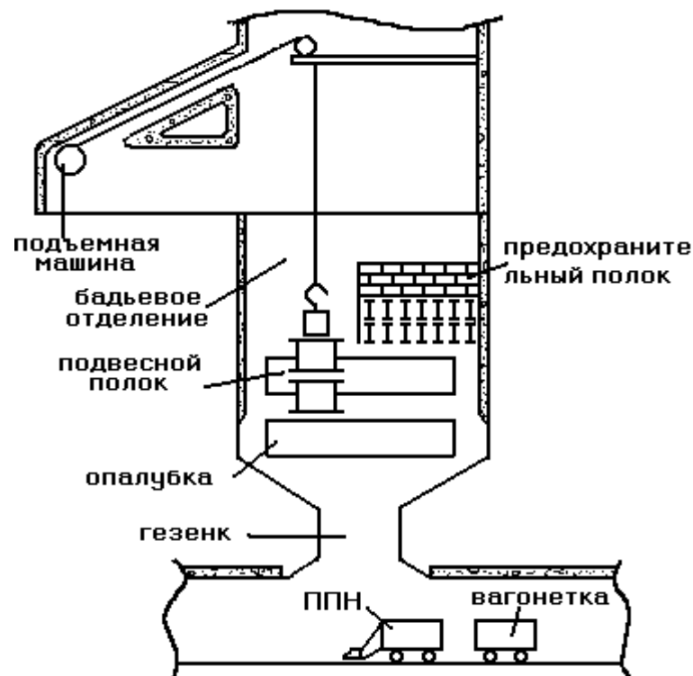
Рисунок 1.4 - Схема углубки ствола комбинированным способом.
