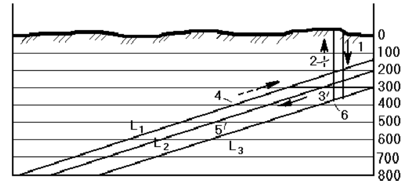
Рисунок 1.1- Исходная схема вскрытия:
