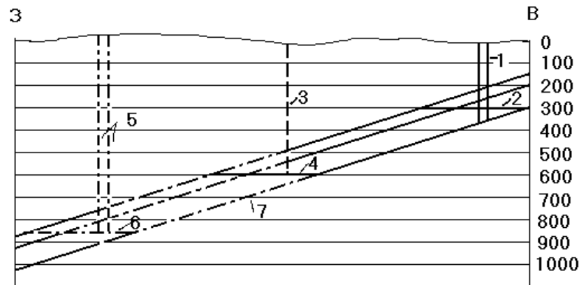
Рисунок 1.2 - Схема вскрытия при реконструкции. Выработки, проведенные на 1 и 2 этапе реконструкции.
