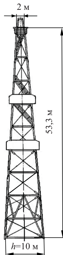
Рис. 1. Общий вид башенной вышки ВБ-53-320
