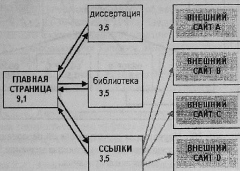
Рисунок 9 – Существующая структура связей типичного персонального сайта портала.
