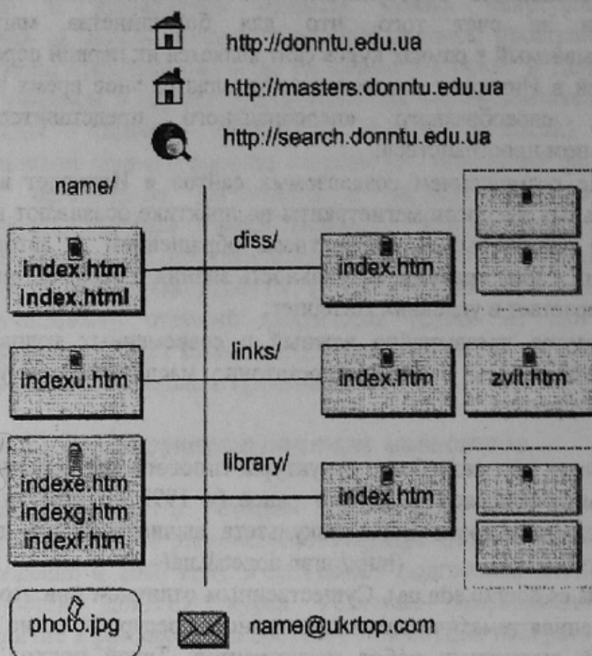
Рисунок 1 – Структура персонального сайта магистра
