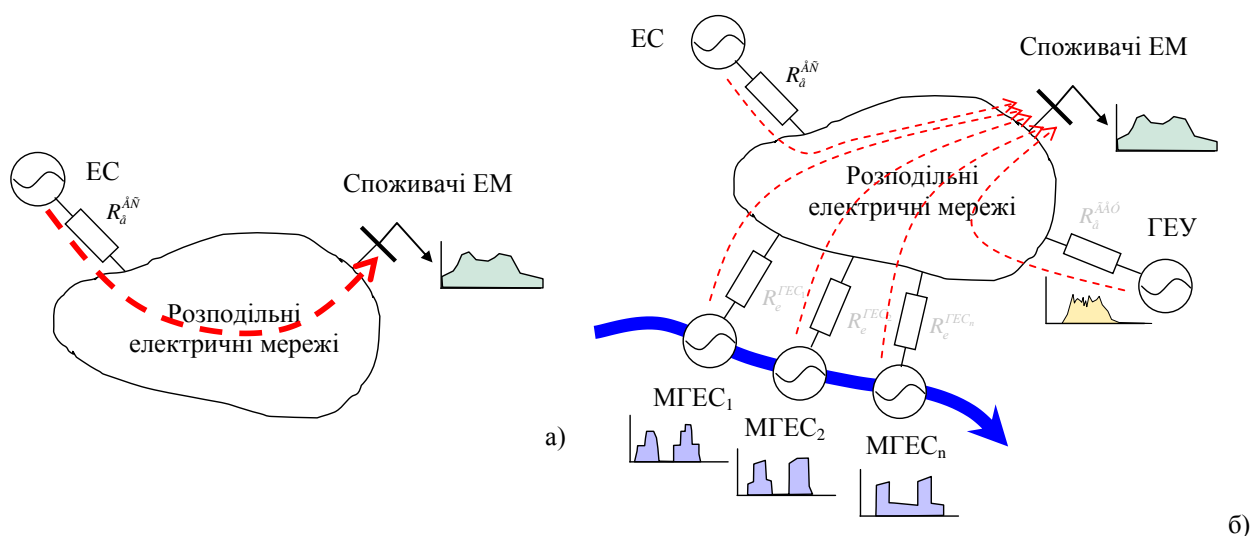
Рисунок 1 - Розподільні електричні мережі з розосередженими джерелами енергії
