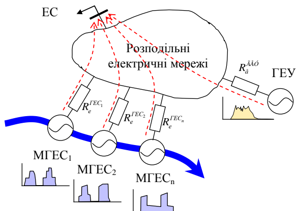
Рисунок 2- Щодо задачі оптимізації функціонування РДЕ в розподільних електричних мережах
