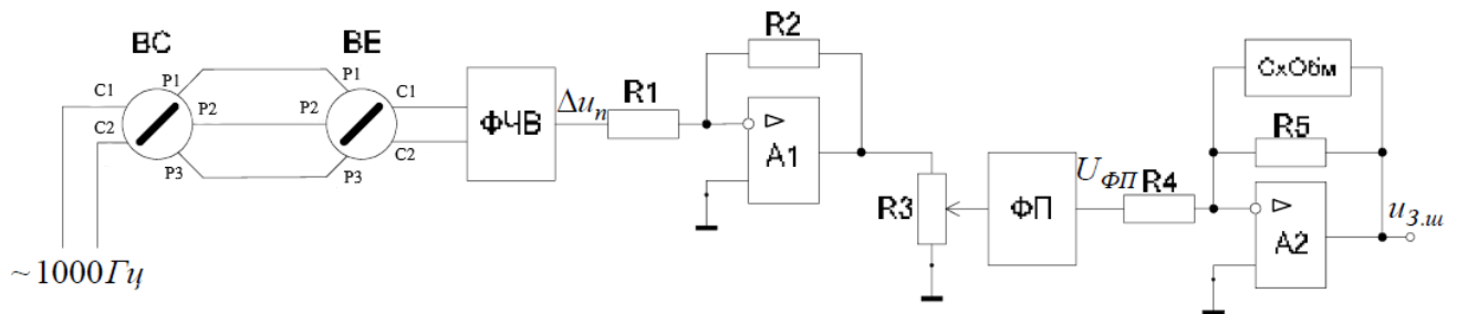
Рисунок 3.14 – Схема аналогової реалізації параболічного РП
