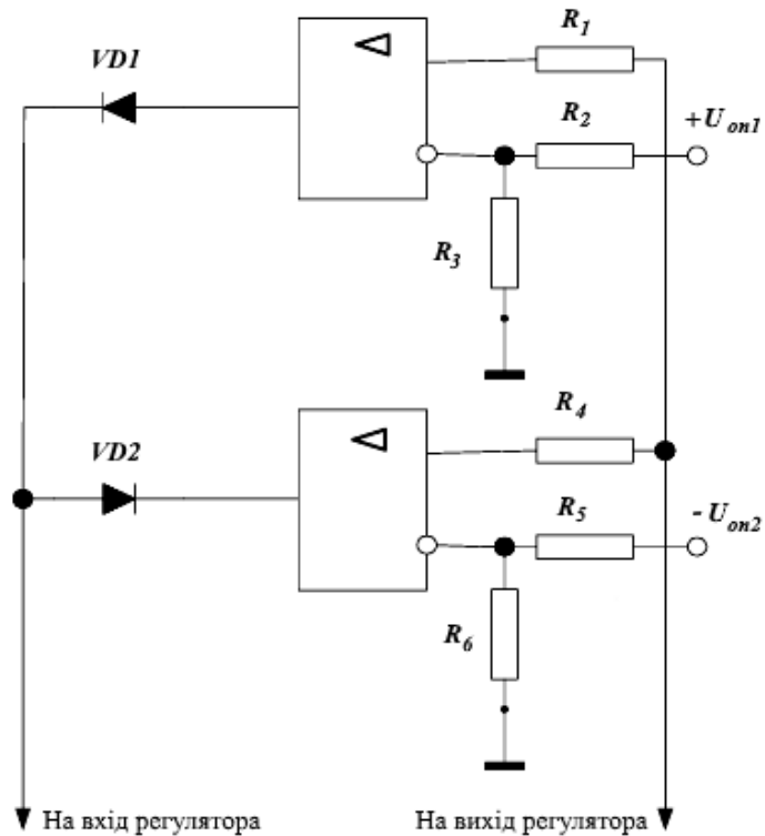
Рисунок 3.11 – Реалізація обмеження вихідної координати
