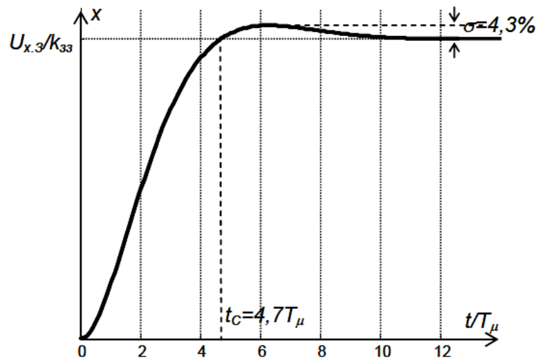
Рисунок 3.7 – Реакція замкненого контуру на стрибок завдання U_{x,3}
