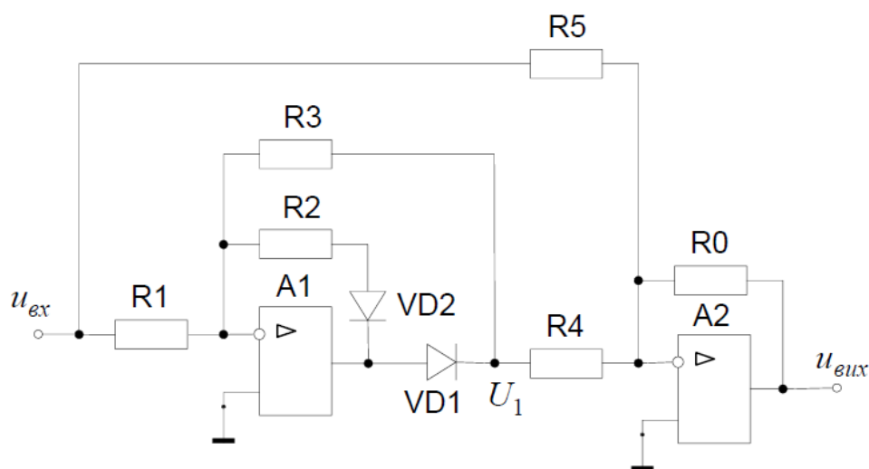
Рисунок 3.13 – Реалізація операції виділення модуля
