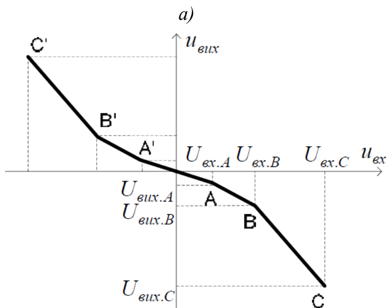
Рисунок 3.12 – Схема реалізації ФП (а) та його характеристика (б)
