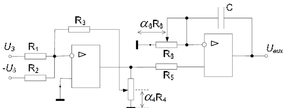
Рисунок 3.10 – Варіант схеми реалізації регулятора швидкості
