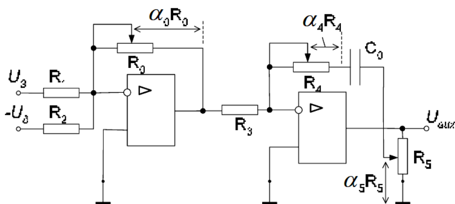
Рисунок 3.9 – Варіант схеми реалізації регулятора струму
