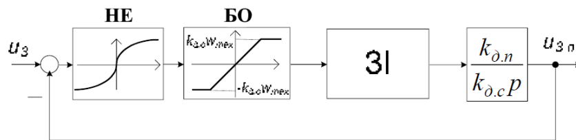
Рисунок 3.16 – Структурна схема задатчика положення
