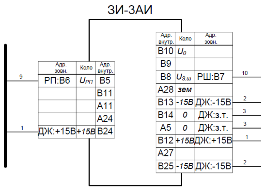
Рисунок 3.17 – Зображення комірки ЗІ-ЗАИ з виводами (на схемі з'єднань)
