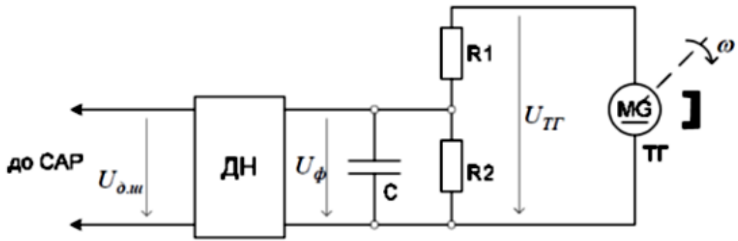
Рисунок 3.5 – Реалізація зворотного зв'язку за швидкістю
