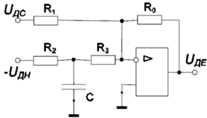
Рисунок 3.4 – Схема реалізації датчика ЕРС
