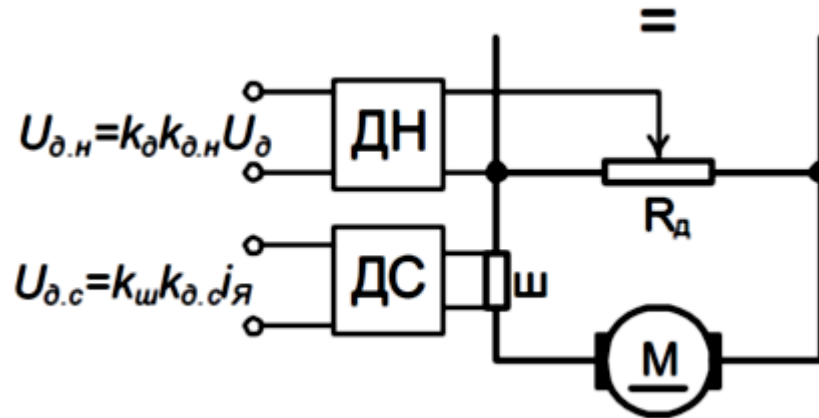
Рисунок 3.3 – Схема вимірювання напруги і струму кола якоря
