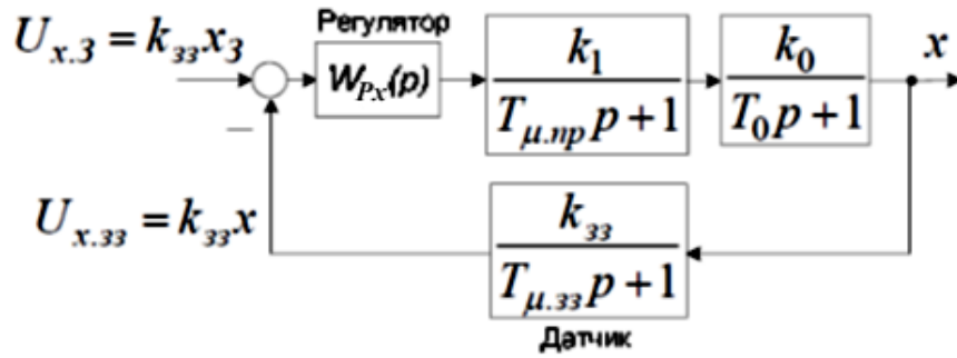
Рисунок 3.6 – Структурна схема контуру регулювання
