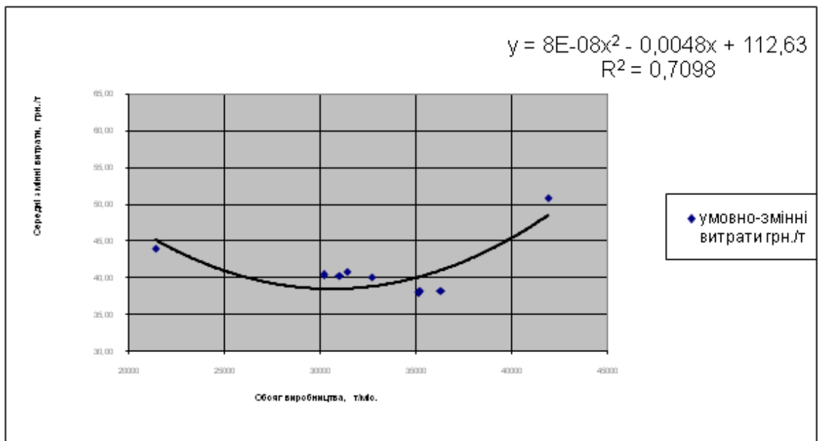
Рисунок 7 – Результат аналізу та вибору рівняння залежності (на прикладі обрання поліному 2-го ступеню)
