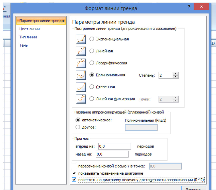
Рисунок 6 – Аналіз та вибір рівняння залежності
