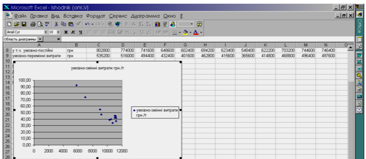
Рисунок 5 - Побудова діаграми та кореляційного поля при визначенні форми залежності
