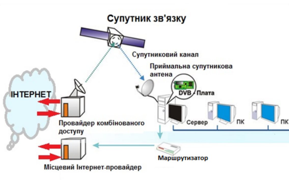
Рисунок 1 – Архітектура гібридної системи супутникового зв'язку
