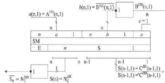
Рисунок 8 – Схема віднімання цілих чисел в коді з додатним нулем
