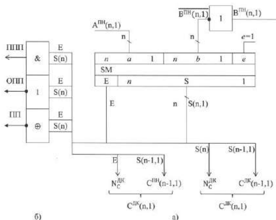
Рисунок 9 – Модифікована схема віднімання цілих чисел в кодах з додатним нулем: а) операційний суматор; б) схема фіксації переповнення
