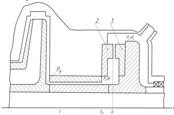
Рисунок 1 – Розвантажувальний пристрій шахтного насоса як механічна коливальна система.
