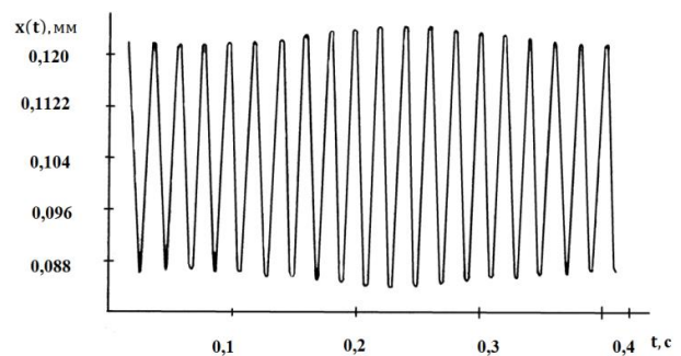
Рисунок 2 – Характеристика коливального процесу ротора насоса.
