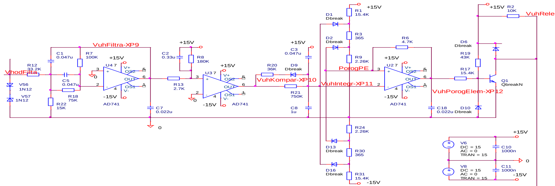
Рисунок 2.2 – B-структура TS. Ненаправлений TS «Час-імпульсний критерій». Принципова схема реле PTZ-51 з новими параметрами для промислової частоти
