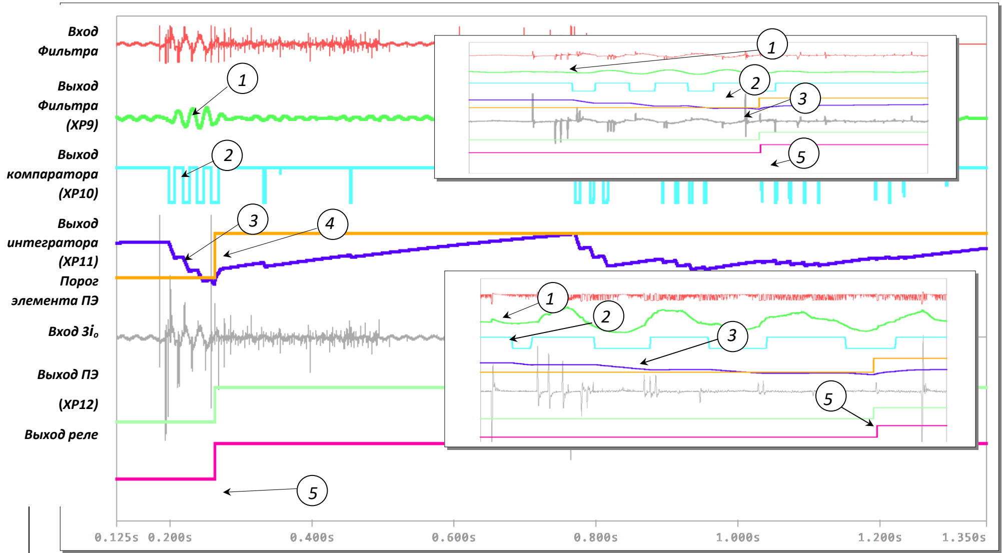
Рисунок 2.3 – Кар'єрна мережа, I_c=4A . «Короткочасне металеве ОЗЗ». Моделювання роботи датчика для J-структури TS з реле PT3-51. Для реального сигналу смислової SN «Короткочасне металеве ОЗЗ». Сигнали для пошкодженої ділянки мережі. Моделювання роботи реле з новими параметрами для промислової частоти. Сигнали пошкодженого ( K_u = 0.000127 ) і неушкодженого приєднань ( K_u = 0.005 ) мережі. Ефективна фільтрація ВЧС Zi_o (див. Т1). Селективне Зведення реле (див. Т2). Час контролю часо-імпульсного критерію роботи реле (див. Т3). Селективне спрацювання порога pN (див. Т4). Правильна видача сигналу про спрацювання реле (див. Т5)
