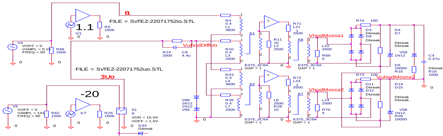
Рисунок 2.1 – I-, J-структура TS. Направлений смарт-TS «1 і 2 ТТНП 3іо з додатковою обмоткою 3іо без реле» з параметрами для промислової частоти
