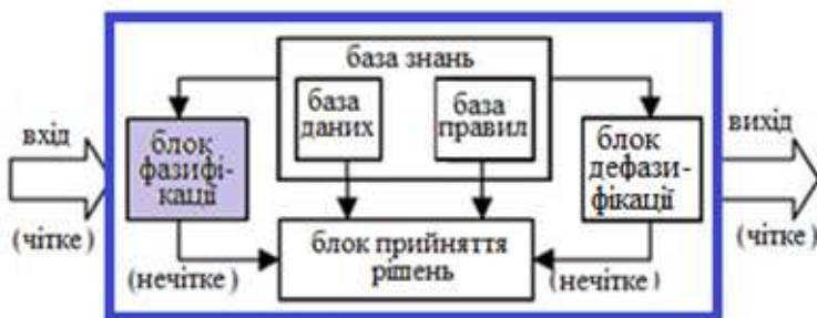
Рис. 1 Схема алгоритму
