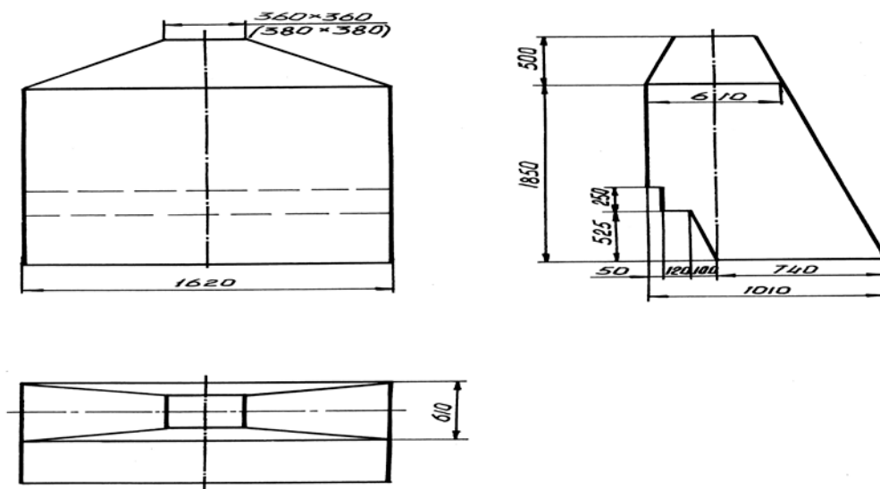
Рис. 1. Местный отсос от загрузочного окна термопечи
