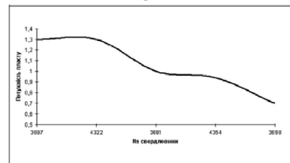
Рис. 5. Графік коливання потужності пласта для північного крила за простяганням
