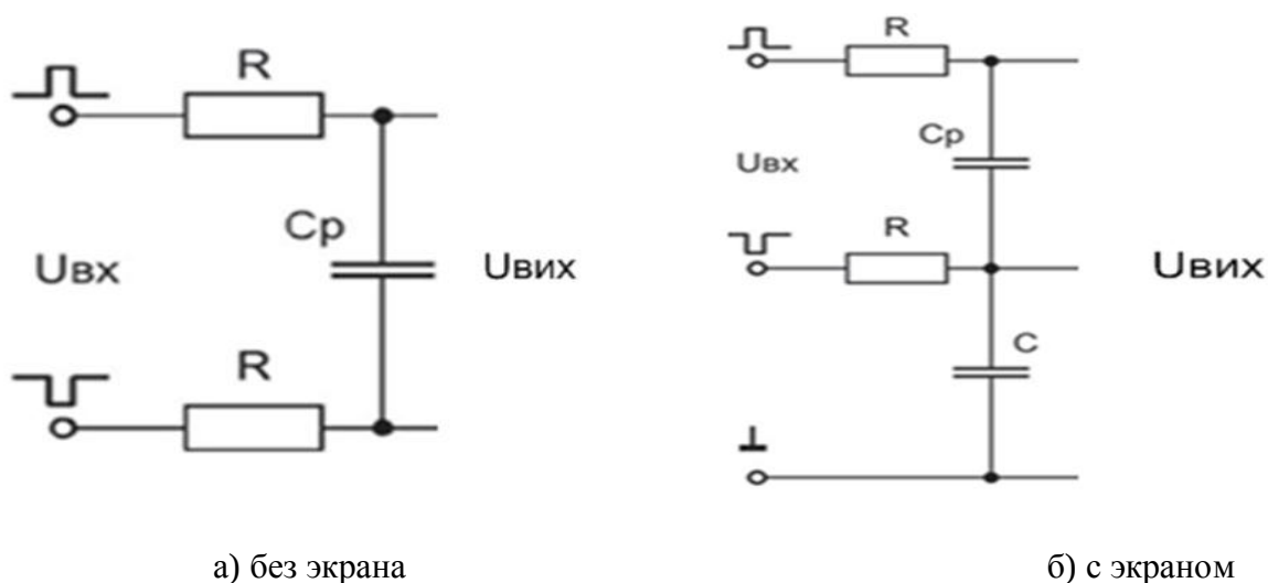
Рисунок 1. Эквивалентная схема замещения длинной линии
