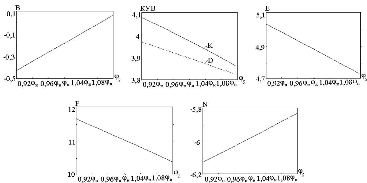
Рисунок 3 - Графіки залежності КУВ при зміні всіх фаз \varphi_s елементів матриці розсіювання СХВ
