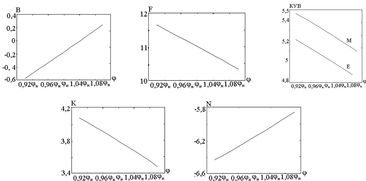
Рисунок 2 - Графіки залежності КУВ СХВ від фаз коефіцієнтів відбиття приймальної антени \varphi_A , еквівалента антени \varphi_R , входів модулятора \varphi_1 і змішувача \varphi_4
