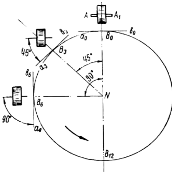
Рис.1 - Отклонение гироскопа с течением времени от плоскости
