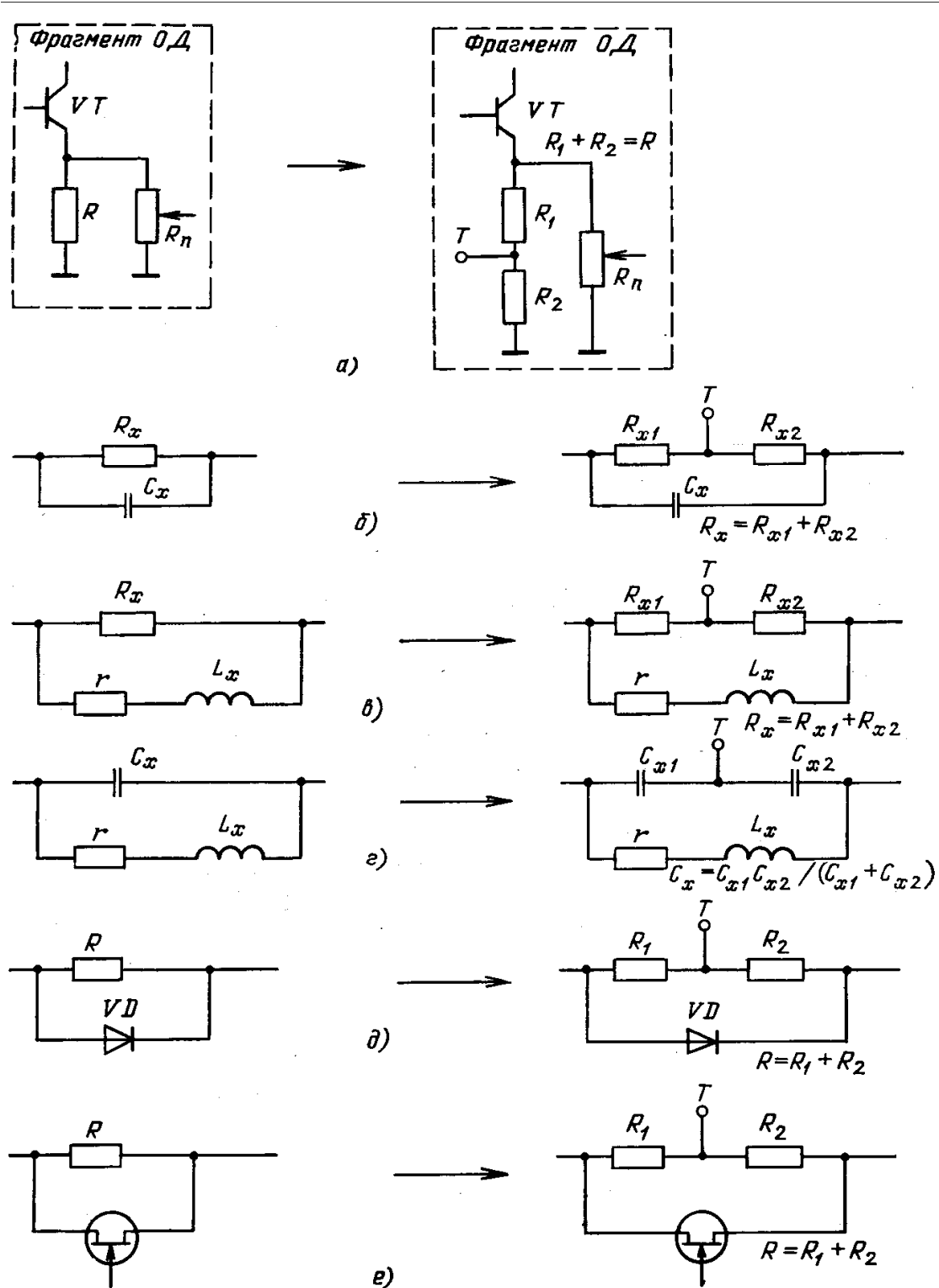
Рисунок 2 — Введення тестових точок для контролю пасивних двополюсників
