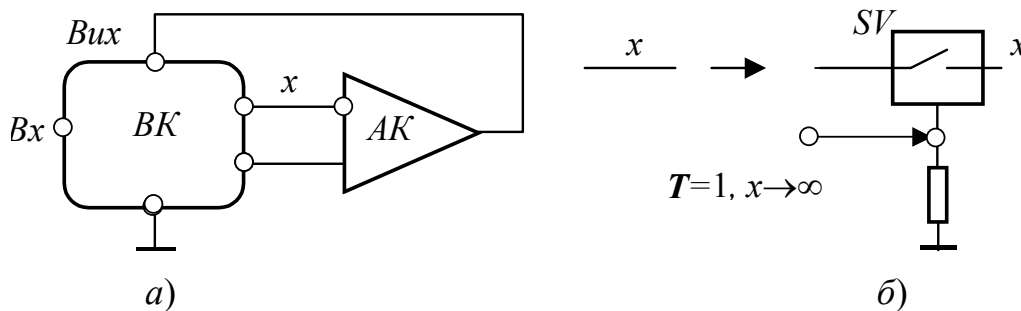
Рисунок 3 — Введення точки T для керованості входу ОП
