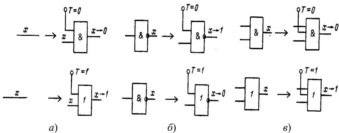
Рисунок 1 — Введення додаткових тестових точок T
