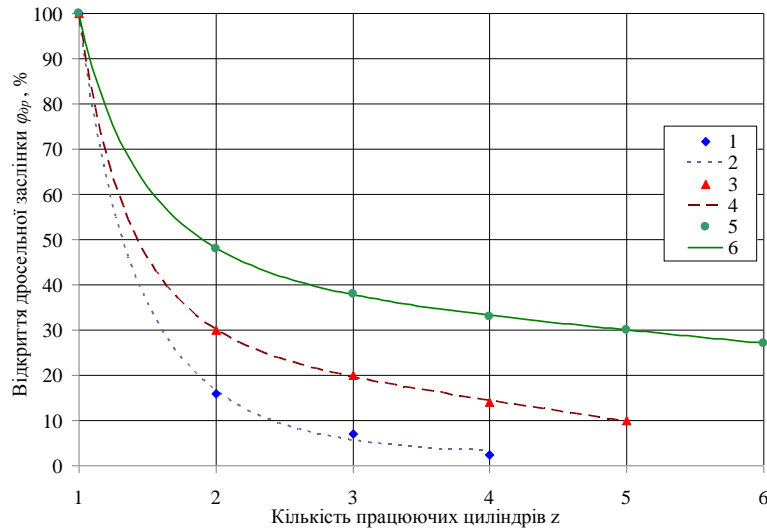
Рисунок 2 – Залежність величини кута відкриття дросельної заслінки \varphi_{др} від кількості працюючих циліндрів z при різних частотах обертання n
