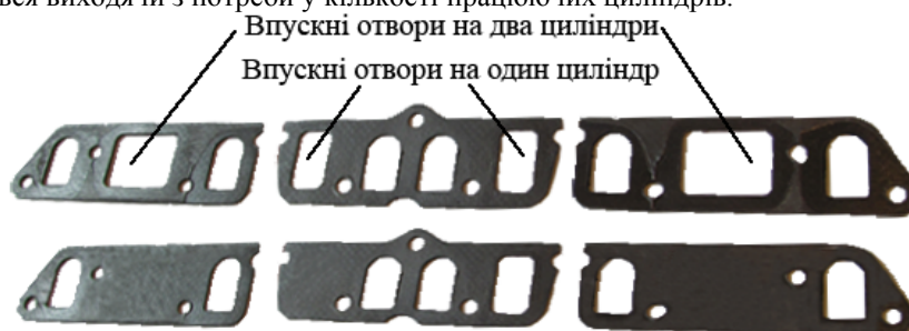
Рисунок 1 – Прокладки газопроводів двигуна ГАЗ-51 Штатні (зверху); використовувані в експерименті (знизу) – один працюючий циліндр
