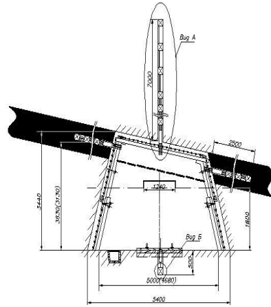
Рис. 3 Общий вид (а) и схема размещения реперов (б) на комплексных измерных станциях в шестом южном конвейерном штреке пласта m_5^{1B} гор. 450 м
