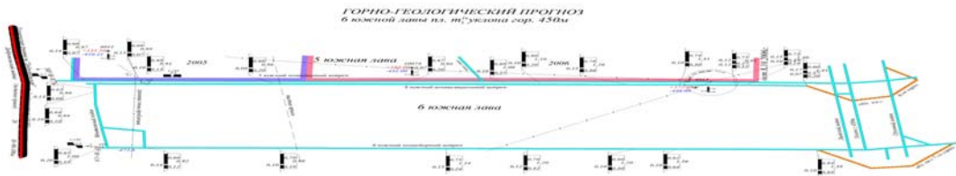
Рис.4 Выкопировка из плана горных выработок по пласту m_5^{1B}
