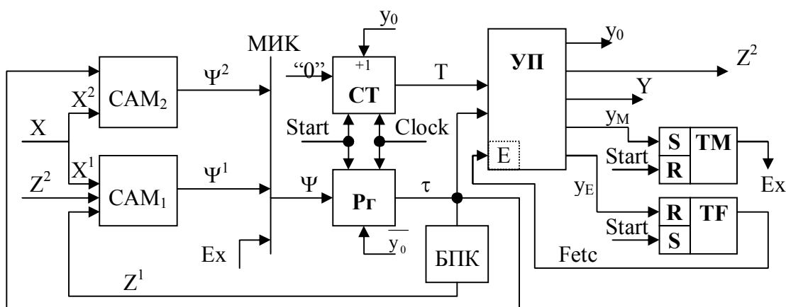
Рисунок 2 – Структурная схема КМУУ U_2
