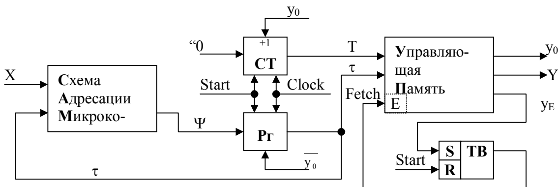
Рисунок 1 – Структурная схема КМУУ с элементарными цепями
